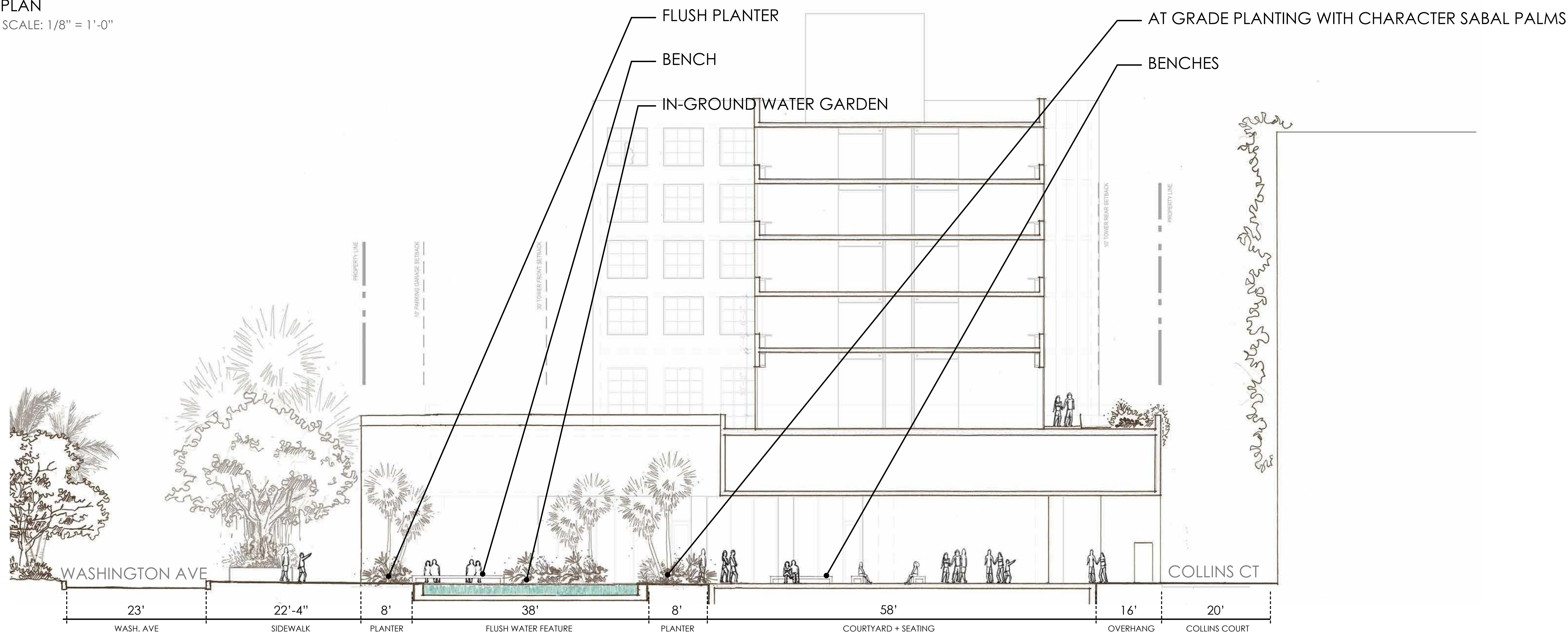
SECTION 5 SCALE: 1/8" = 1'-0"
