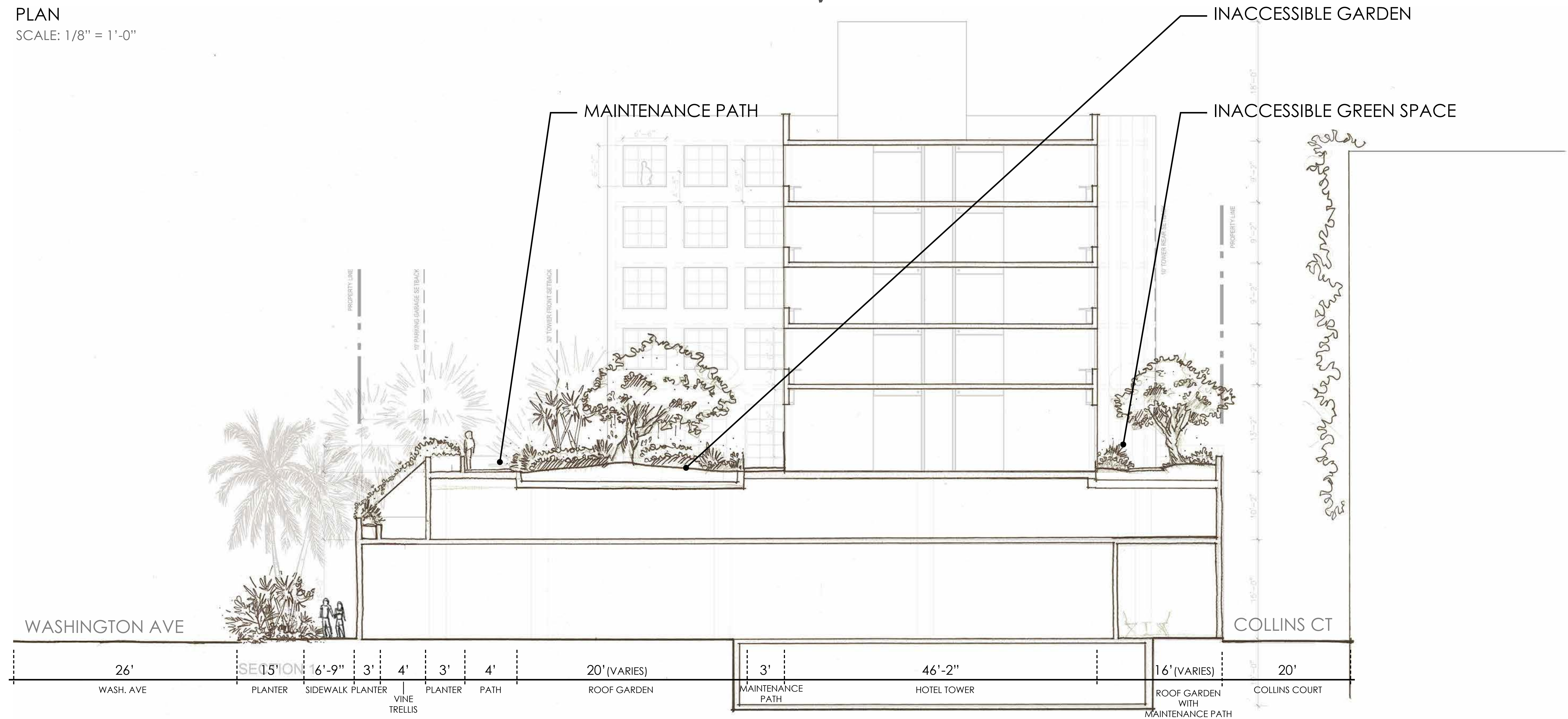
SECTION 6 SCALE: 1/8" = 1'-0"
