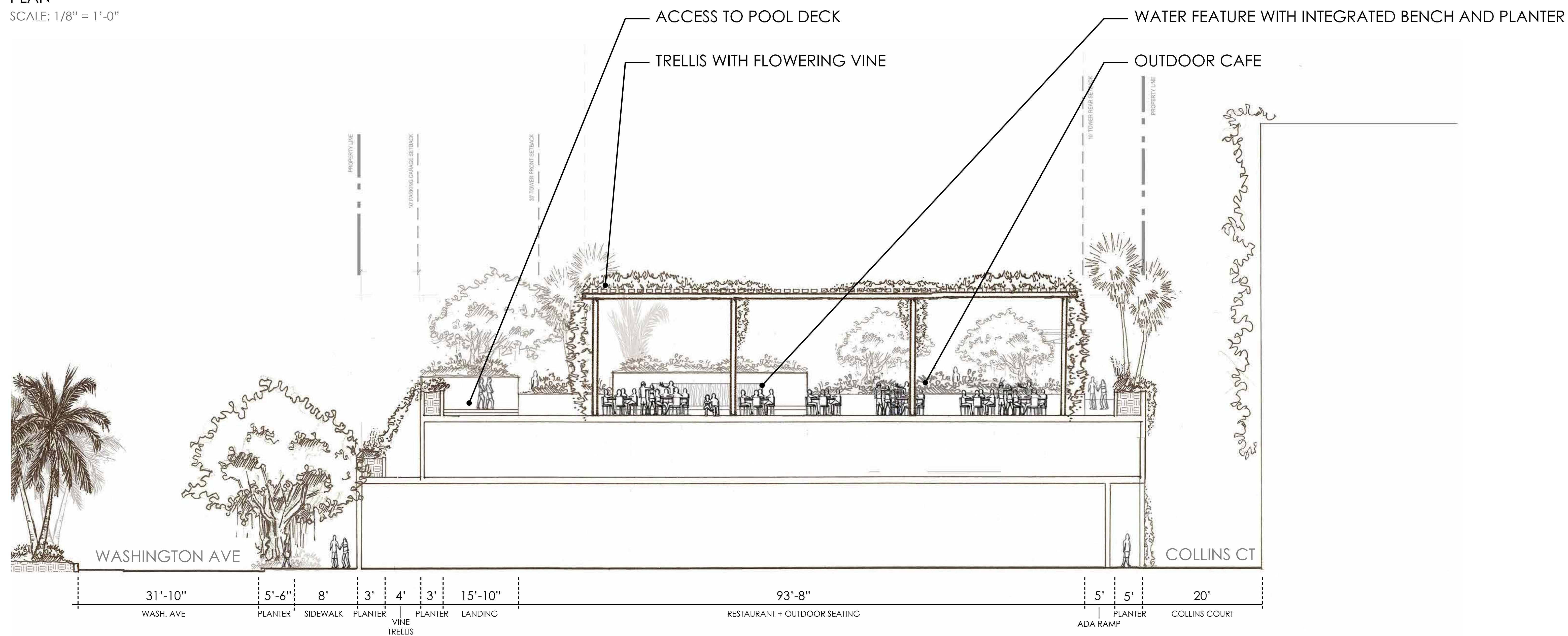
SECTION 4 SCALE: 1/8" = 1'-0"
