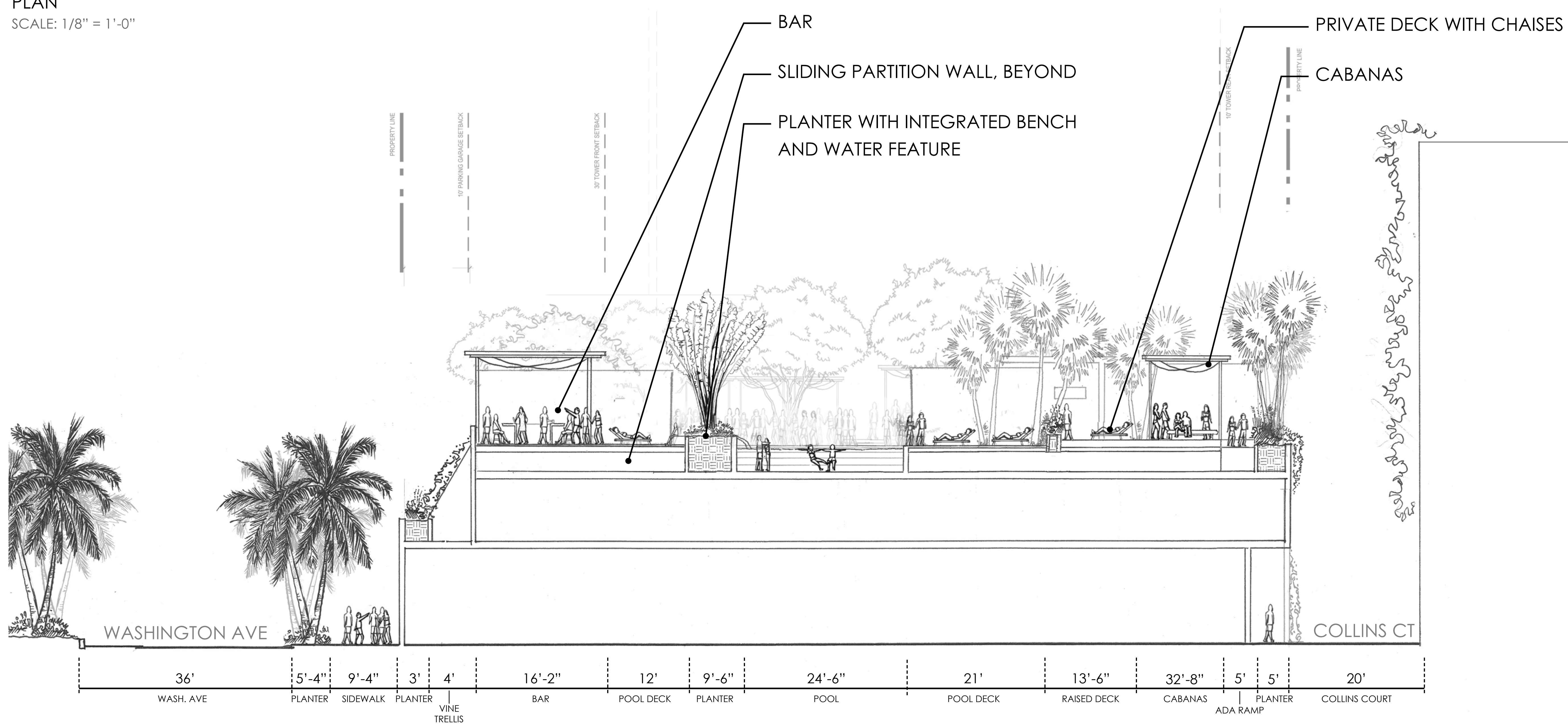
SECTION 2 SCALE: 1/8" = 1'-0"
