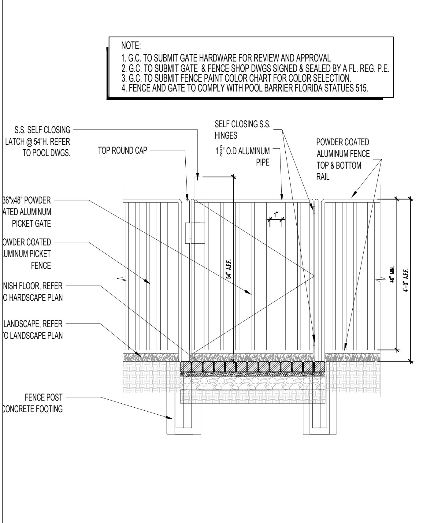
5 GATE DETAIL SCALE: N.T.S.
